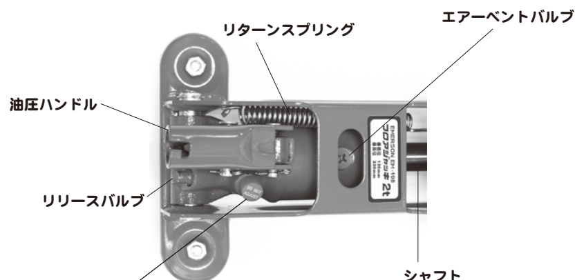
シリンダー部分拡大図
